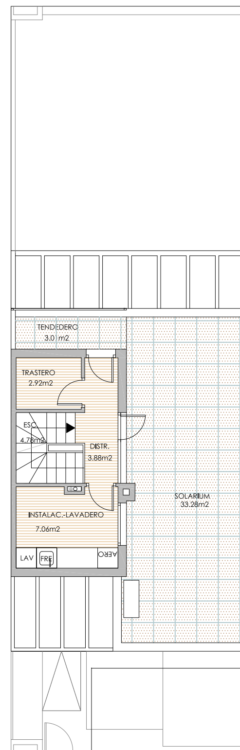
PLANTA CUBIERTA TIPO 3 PLTAS
