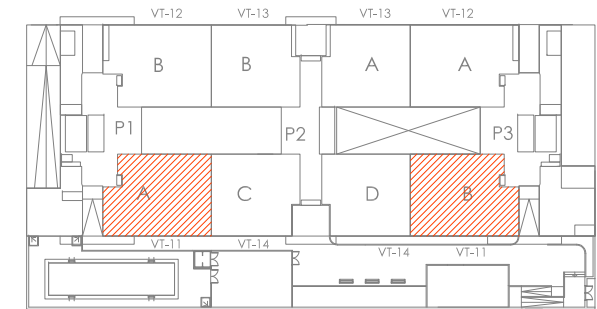
PLANTA BAJA
